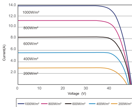
I-V CURVES OF PV MODULE(565W)
