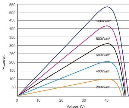
P-V CURVES OF PV MODULE(565W)
